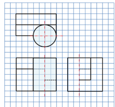
正面図
